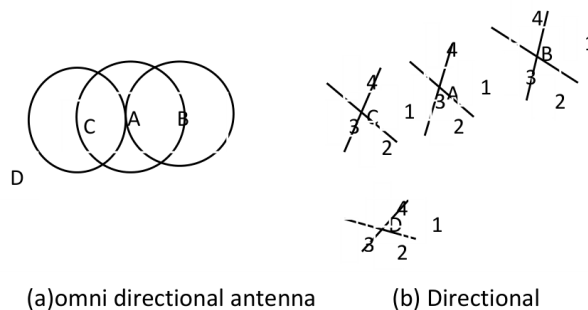
Fig 5: Spatial reuse
